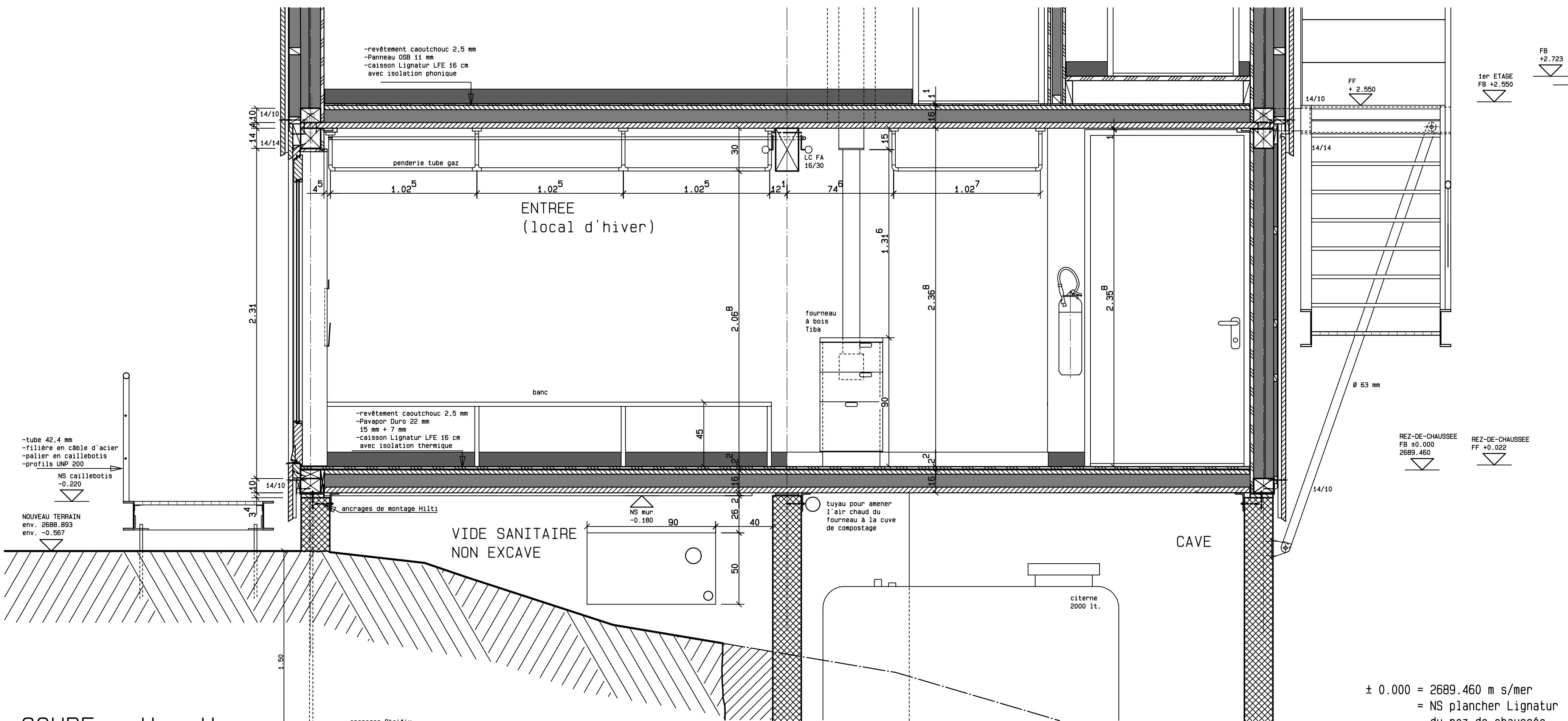
COUPE H - H
