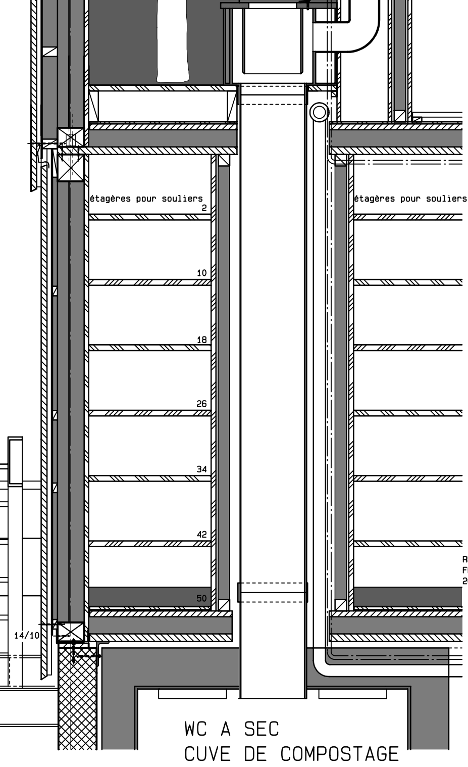
COUPE SUR WC GARDIENS
