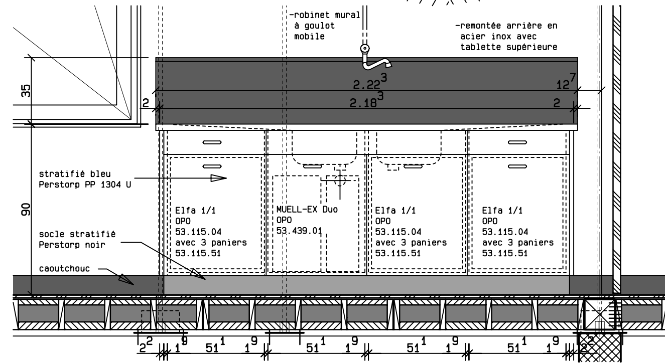
COUPE N - N
