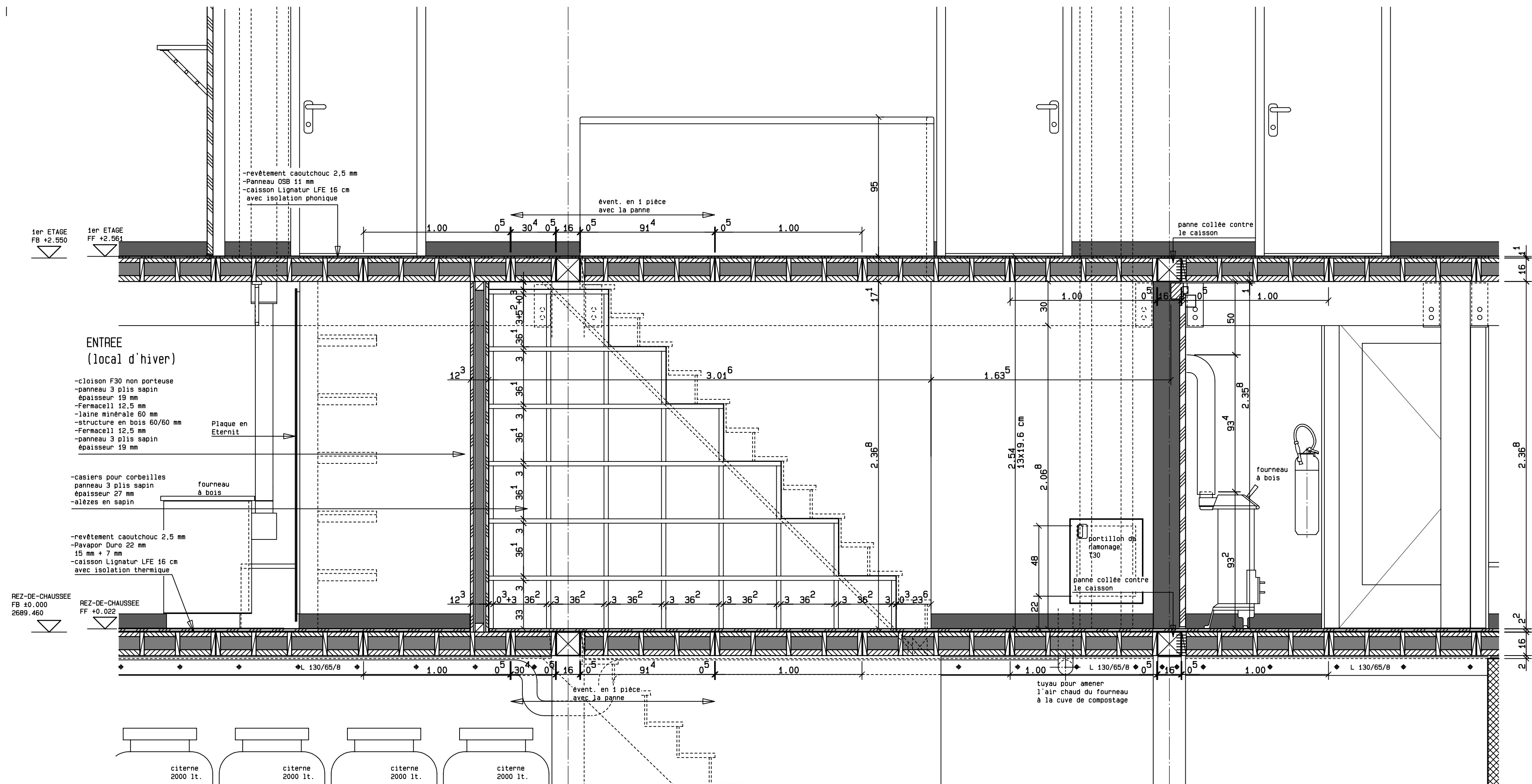
COUPE F - F casiers
