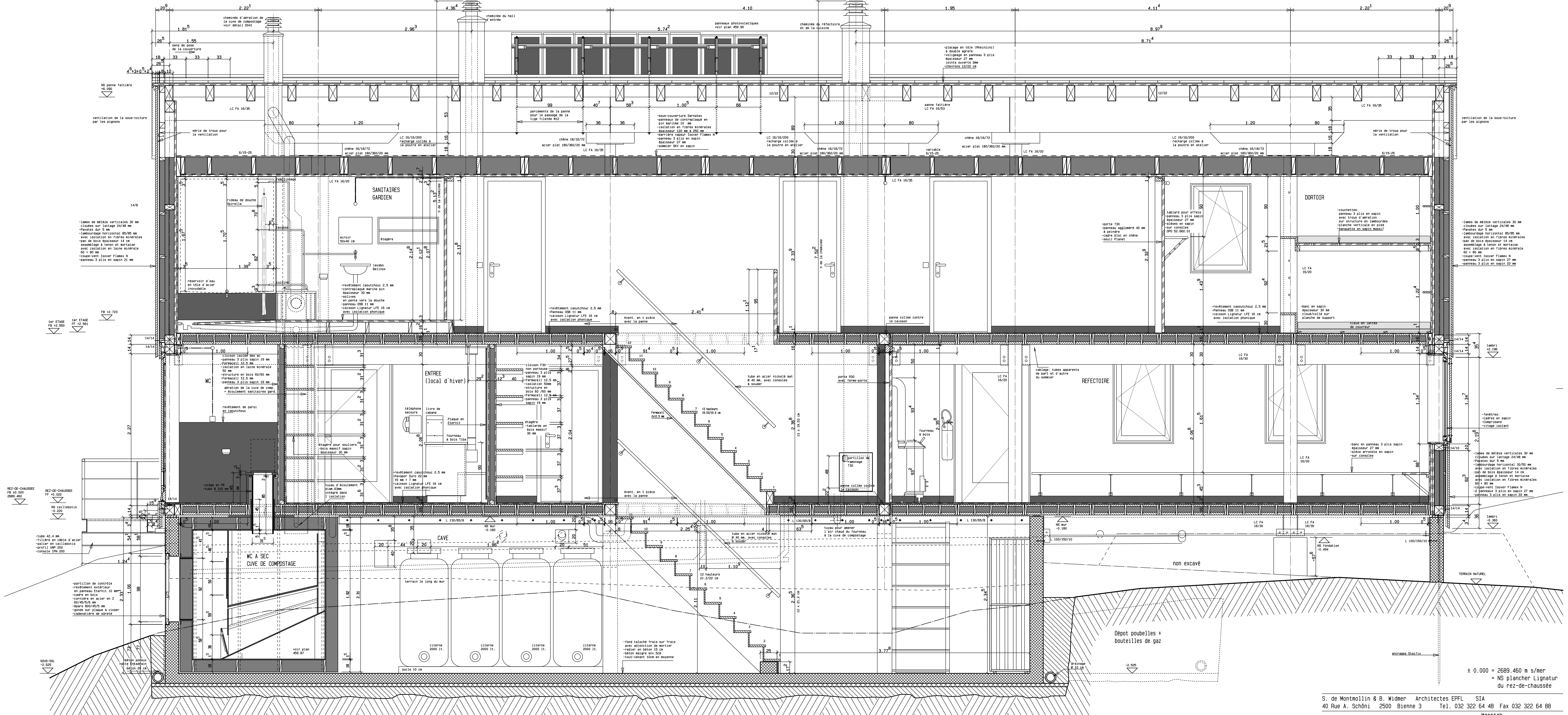
COUPE A - A
